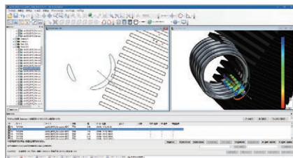
干渉・クリアランスの検出結果
